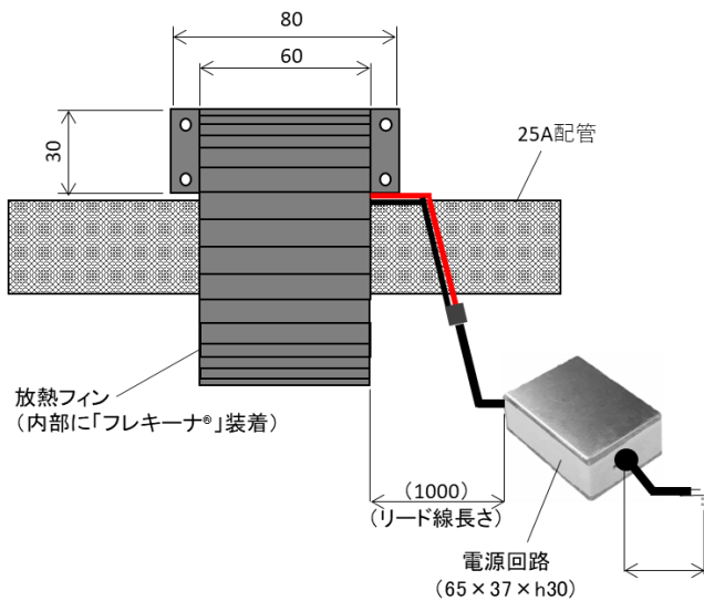
(配管断面図)
